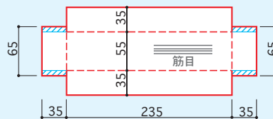
▼個装用トレイ (たばこ10個装填)
